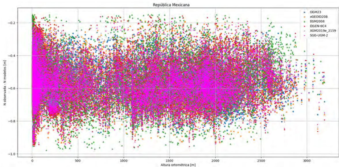
Figura 29. Dispersión de las alturas del geoide calculadas en relación con las alturas ortométricas del lugar con datos de toda la República Mexicana.
