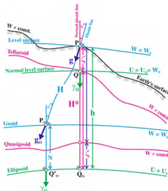
Figura 14. Alturas y superficies de referencia (Sánchez et al., 2021).
