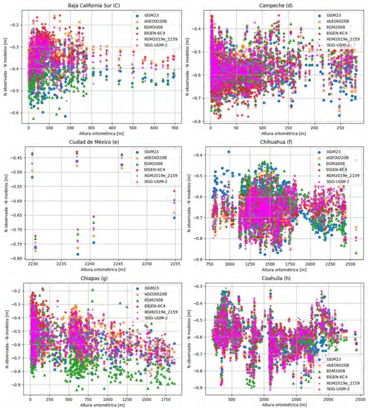
Figura 31. Dispersión de las alturas del geoide calculadas con relación a las alturas ortométricas de Baja California Sur (c), Campeche (d), Ciudad de México (e), Chihuahua (f), Chiapas (g), Coahuila(h).
