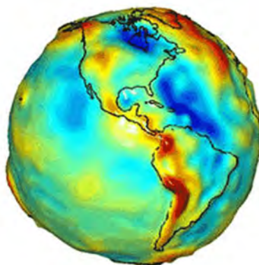
Figura 3. Geoide. Recuperado de https://photojournal.jpl.nasa.gov/jpegMod/PIA12104_modest.jpg .
