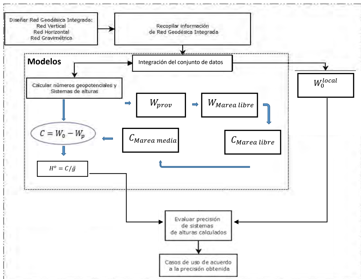
Figura 13. Esquema metodológico.
