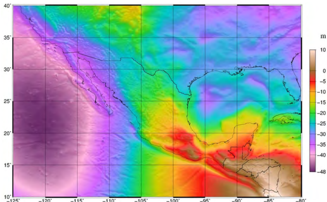
Figura 21. Modelo del Geoide experimental xGGM23 (Avalos-Naranjo, 2024).
