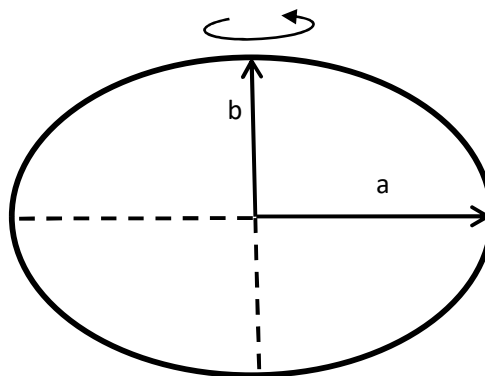
Figura 2. Elipsoide.
