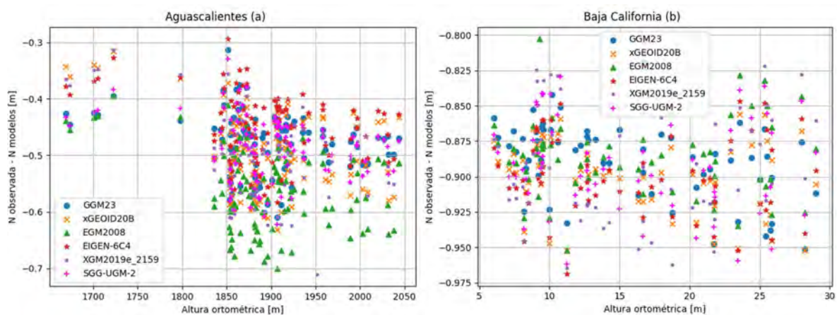
Figura 30. Dispersión de las alturas del geoide calculadas con relación a las alturas ortométricas de Aguascalientes (a), Baja California (b).
