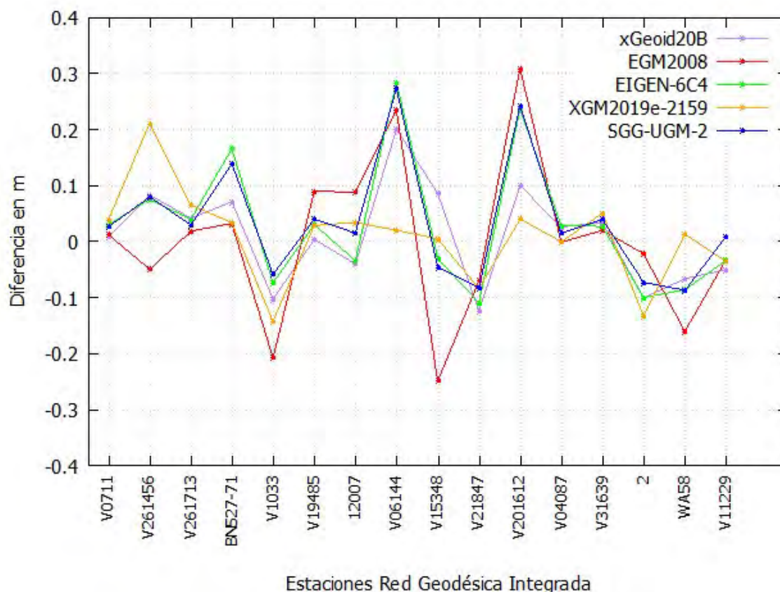
Figura 23. Variación alturas ortométricas de vértices de la Red Geodésica Integrada derivada de modelos respecto al geoide gravimétrico xGGM23.
