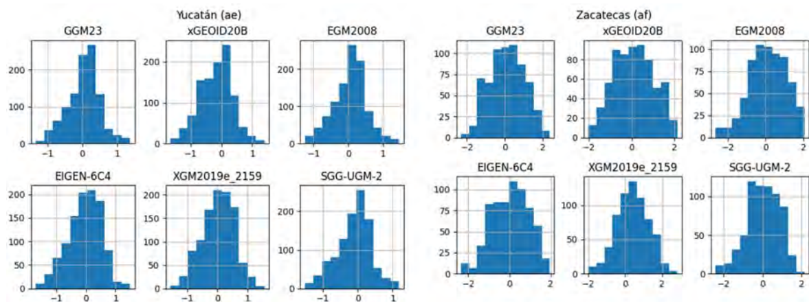
Figura 41. Histogramas de distribución de los datos utilizados en el cálculo del sesgo entre el datum vertical global y local de Yucatán (ae), Zacatecas (af).
