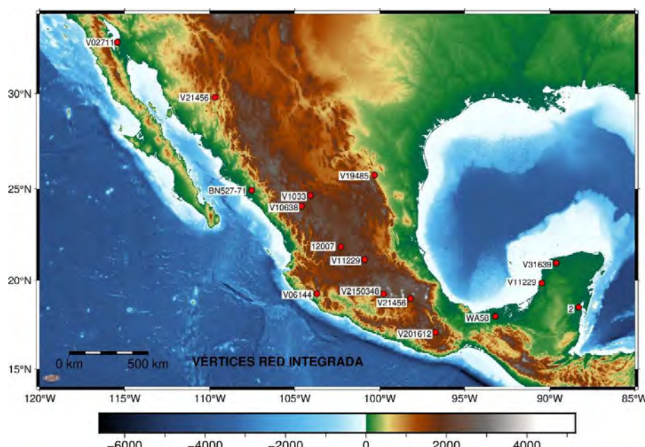
Figura 17. Vértices geodésicos de la Red Geodésica Nacional seleccionados.
