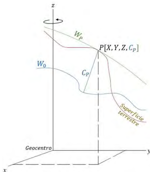
Figura 10. Definición y propuesta de realización del Sistema Internacional de Referencia de Alturas (Sánchez L, 2020)
