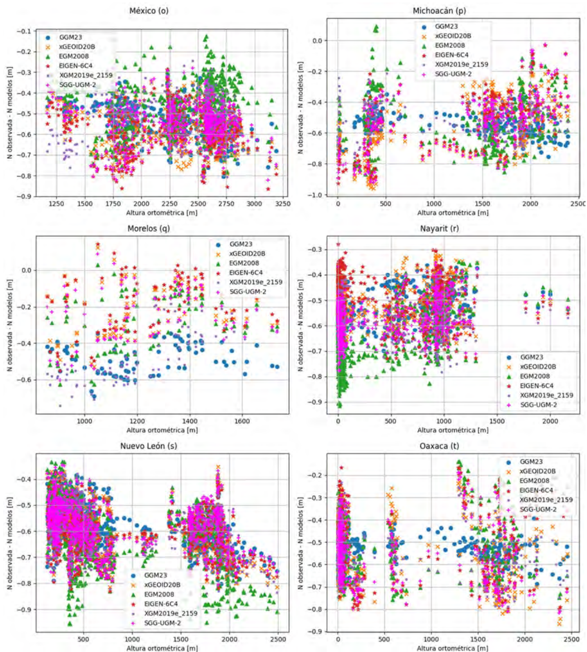
Figura 33. Dispersión de las alturas del geoide calculadas con relación a las alturas ortométricas de México (o), Michoacán (p), Morelos (q), Nayarit (r), Nuevo León (s), Oaxaca (t).
