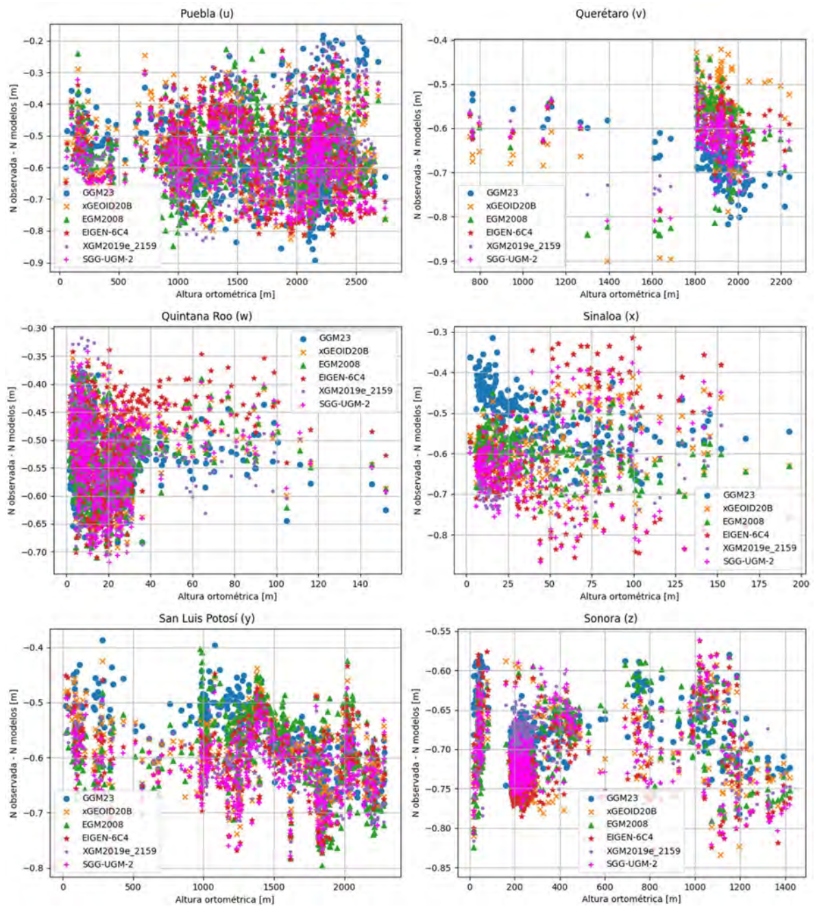
Figura 34. Dispersión de las alturas del geoide calculadas con relación a las alturas ortométricas de Puebla (u), Querétaro (v), Quintana Roo (w), Sinaloa(x), San Luis Potosí (y), Sonora (z).
