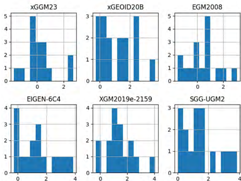
Figura 25. Histogramas de distribución de los datos de la Red Geodésica Integrada utilizados en el cálculo del sesgo entre el datum vertical global y local.
