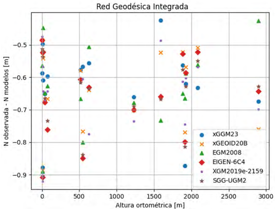
Figura 24. Dispersión de las alturas del geoide calculadas y los diferentes modelos del geoide analizados.
