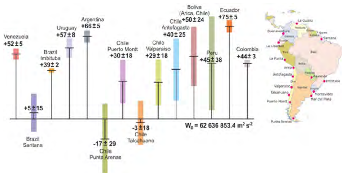
Figura 8. Discrepancias entre datums locales en América del Sur y valor geopotencial de referencia ( W_0 ) (Sánchez & Sideris, 2017).
