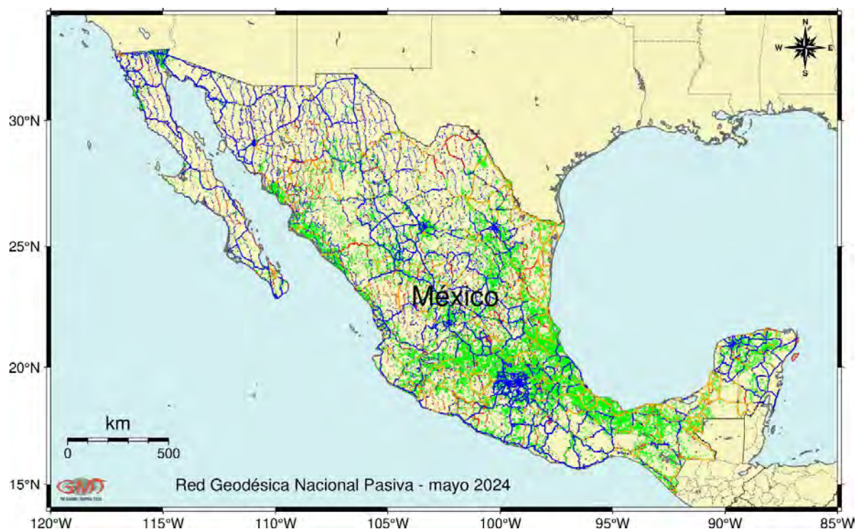
Figura 26. Vértices de la Red Geodésica Nacional Pasiva.
